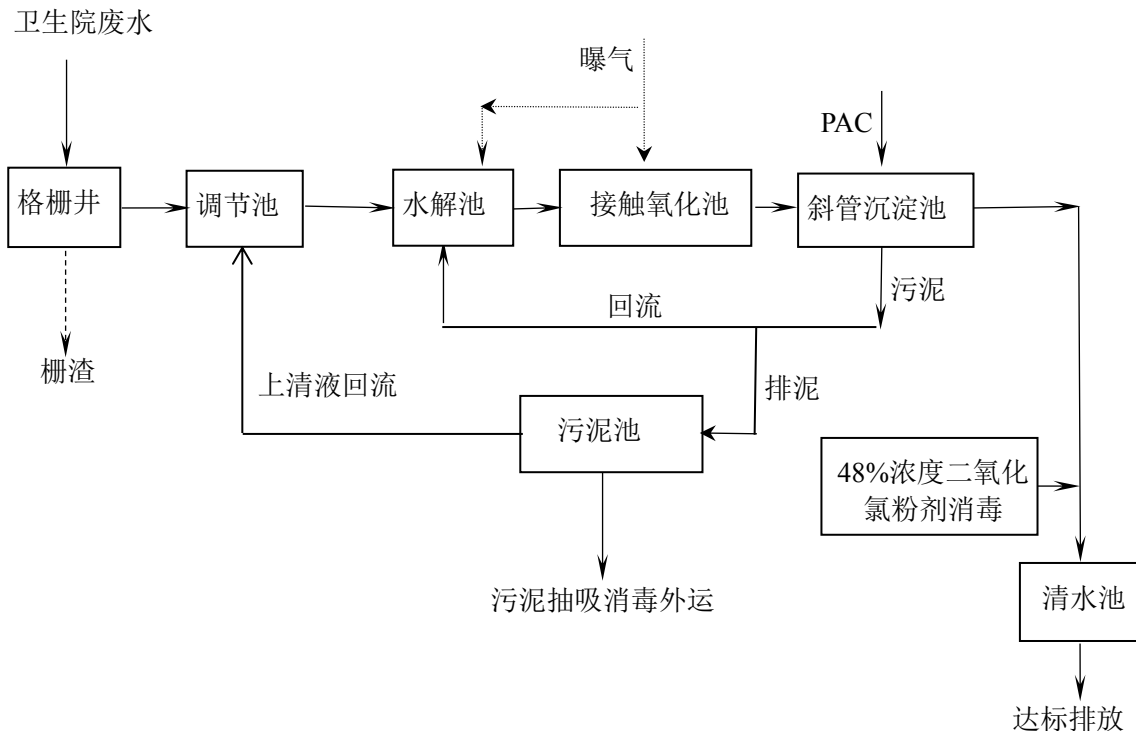
图 4-1 新街镇卫生院污水处理站工艺流程图
