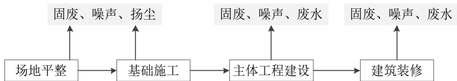
图 3-2 施工期工艺流程及产污节点图
